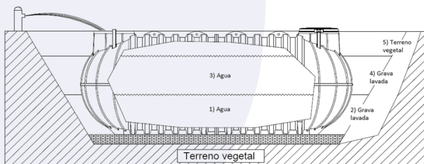
FICHA TÉCNICA: DEPÓSITO EXTERIOR MODELO VERTICAL REFORZADO Ilustración II: Capas de relleno a distribuir para el soterramiento del equipo.
