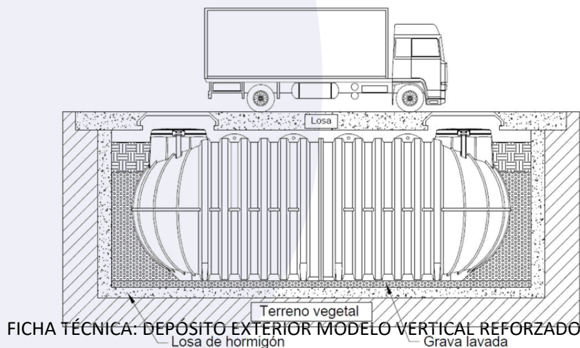
Ilustración XI: Los de HA con encofrado para cargabilidad pesada.
